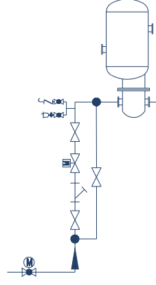
温控阀组
