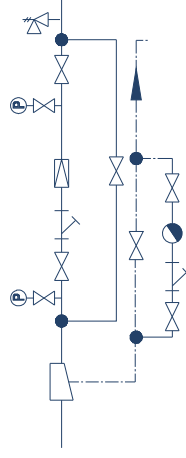
减压阀组
